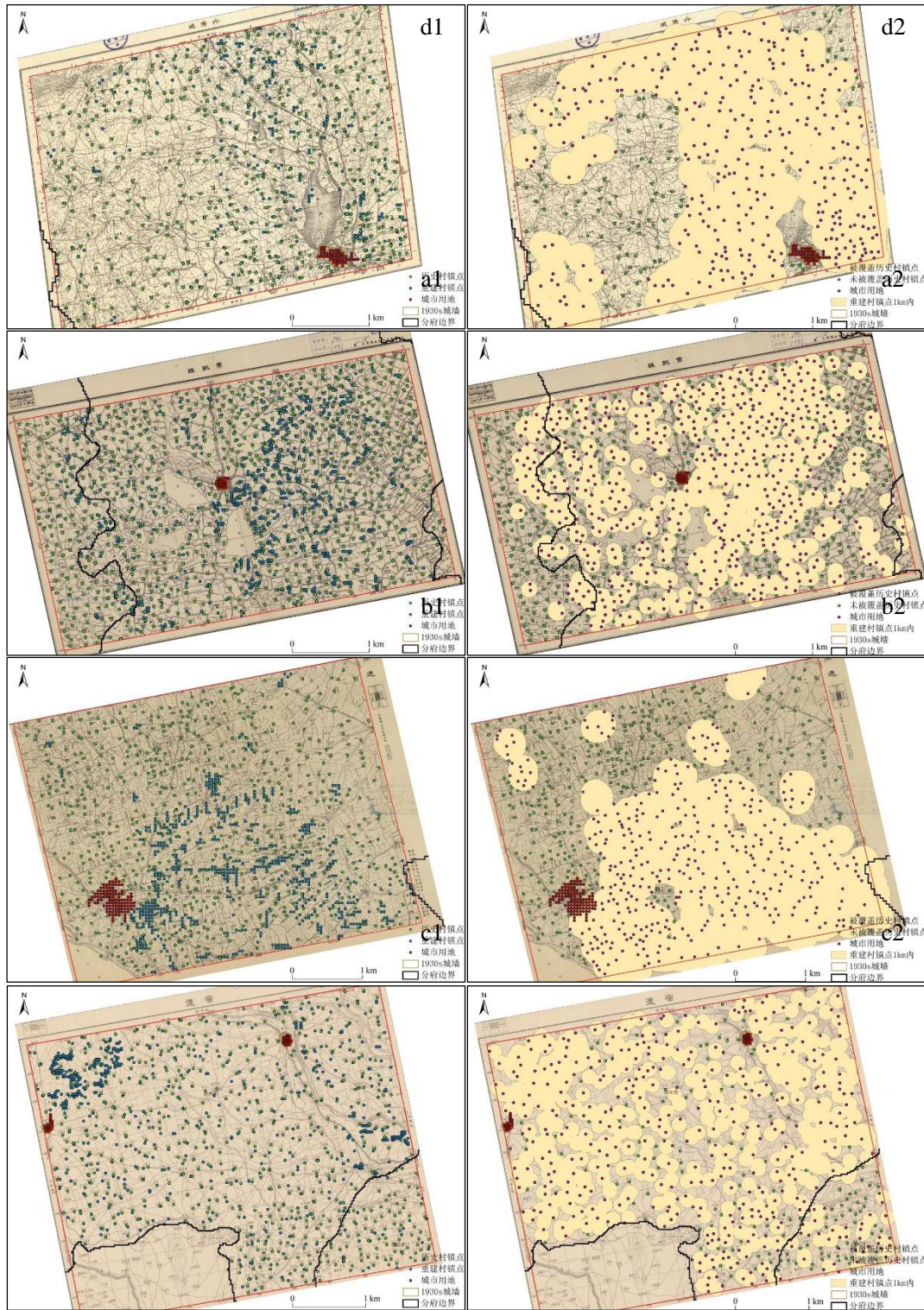
图 7 典型区历史地图(1930s)与重建结果(1936)评估结果
