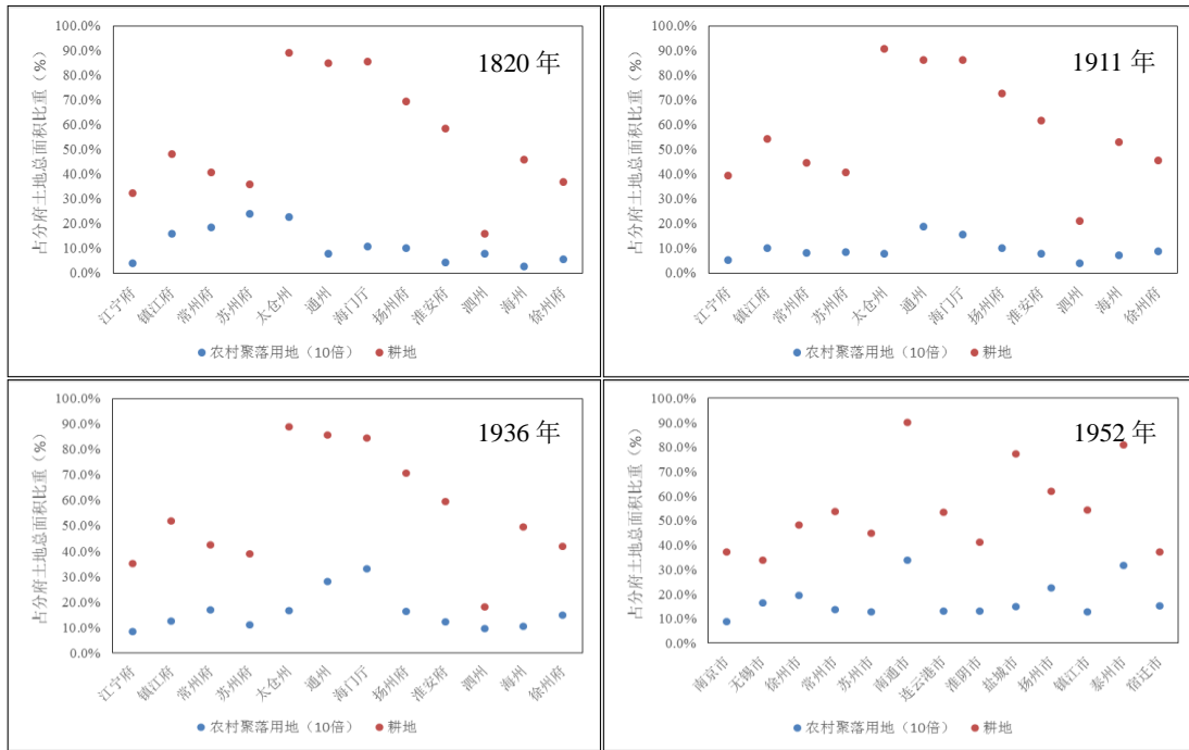
图 6 典型时段分府农村聚落用地与耕地占比
