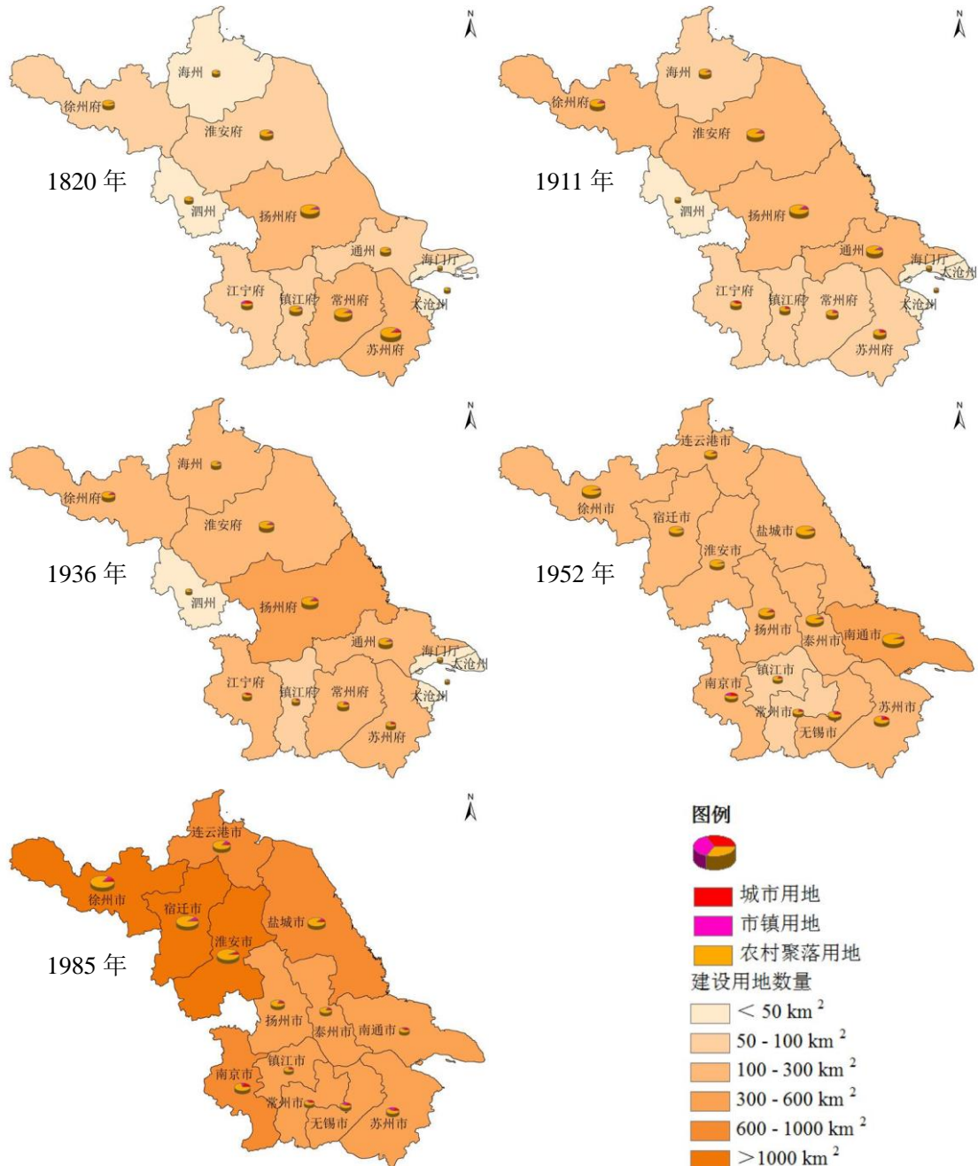
图 3 近 200 年江苏省历史典型时段分府（市）城镇村用地数量变化 Fig.3 Quantity of construction land of Jiangsu in the past 200 years
