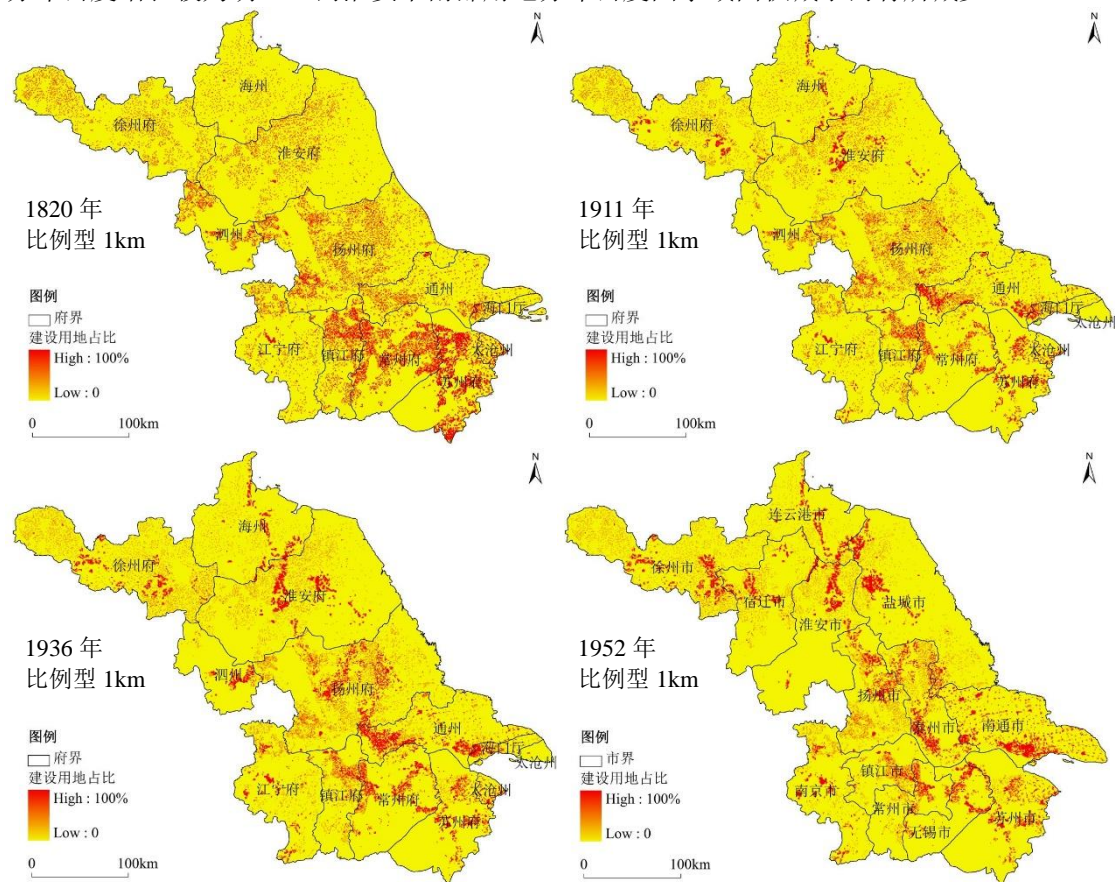
图 5 典型时段江苏省建设用地分布格局
